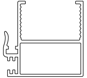
NW-3641 449 gr/mt Takviyeli Çekme Çıta
