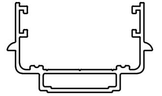
NW-3640 463 gr/mt Bağlantı Adaptör
