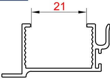
NW-3265 314 gr/mt Tırnaklı Çekme Çıta
